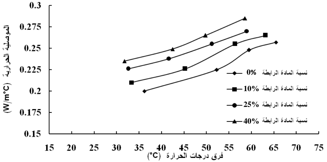
الشكل (8) يبين العلاقة بين الفرق في درجات الحرارة و الموصلية الحرارية.
