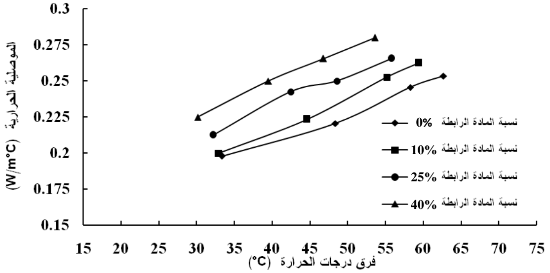
الشكل (7) يبين العلاقة بين الفرق في درجات الحرارة و الموصلية الحرارية.
