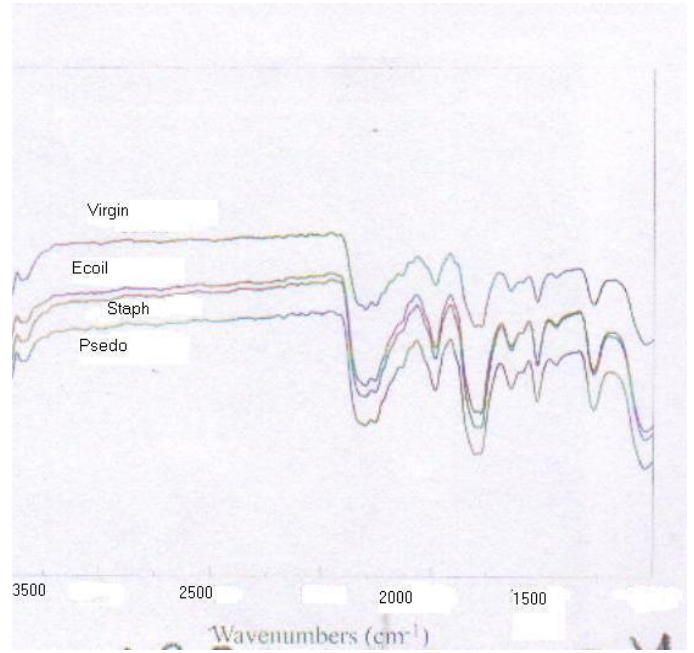
شكل رقم (3) طيف IR لنموذج PVC بين مط OH
