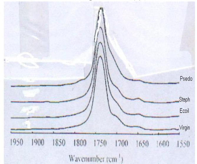
شكل رقم (4) طيف FTIR لنموذج PE بين مط CO
