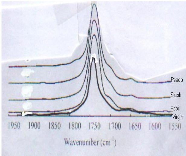
شكل رقم (6) طيف FTIR لنموذج PVC بين مط CO
