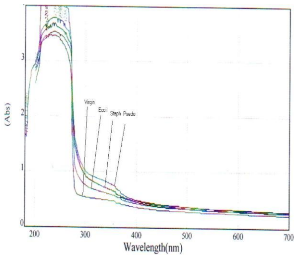
شكل رقم (7) طيف UV لنموذج PE بعد 52 من التعرض للبكتريا
