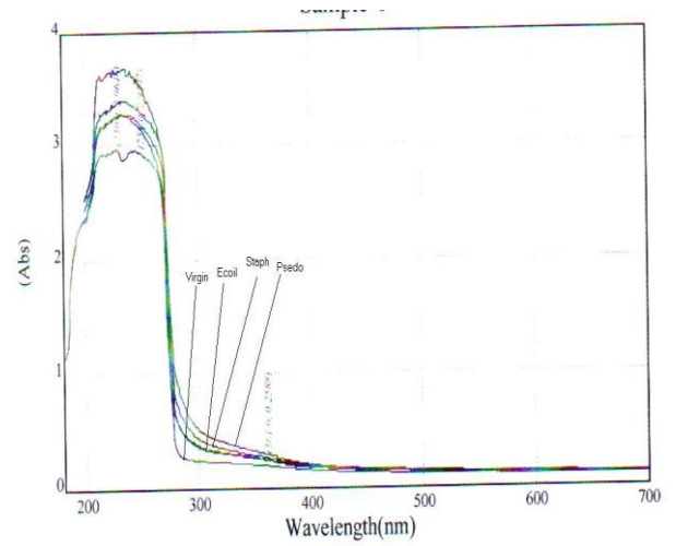
شكل رقم (9) طيف UV لنموذج PVC بعد 52 من التعرض للبكتيريا
