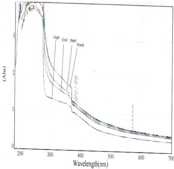
شكل رقم (7) طيف UV لنموذج PE بعد 52 من التعرض للبكتريا
